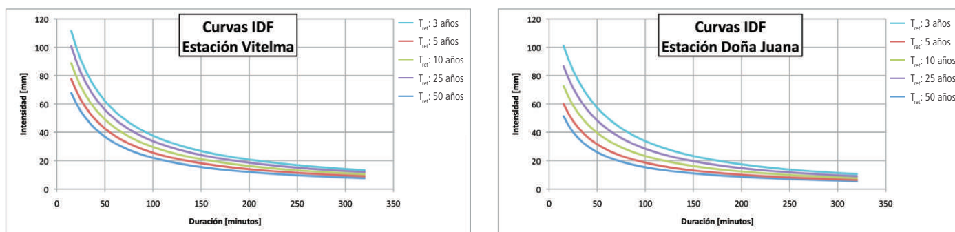
Gráfico 2.4 Curvas típicas de intensidad-duración-frecuencia (IDF)
