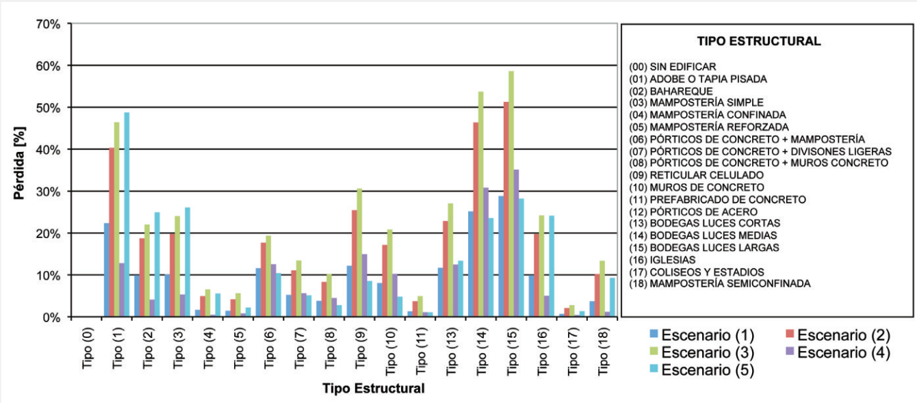
Gráfico 7.8.1 Pérdidas por sistema estructural para el escenario sísmico
