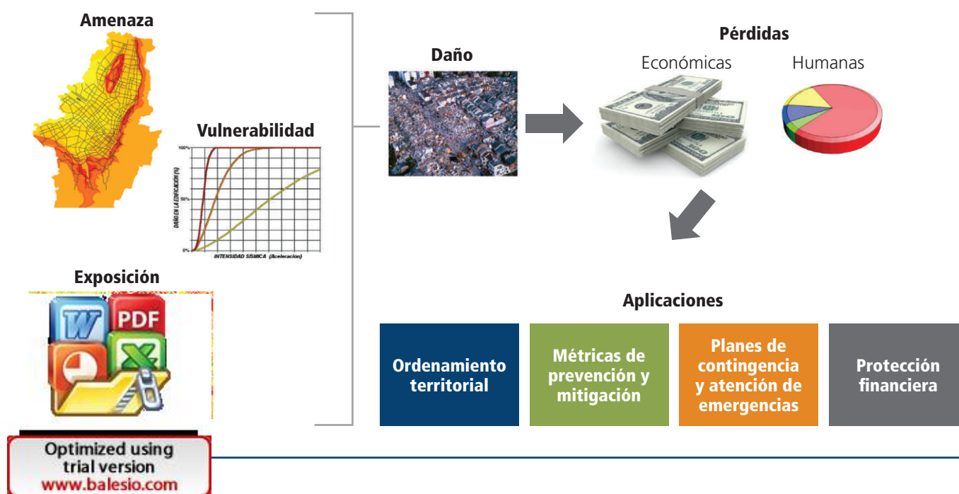
Gráfico 1.2 Esquema del proceso para la evaluación rigurosa del riesgo
