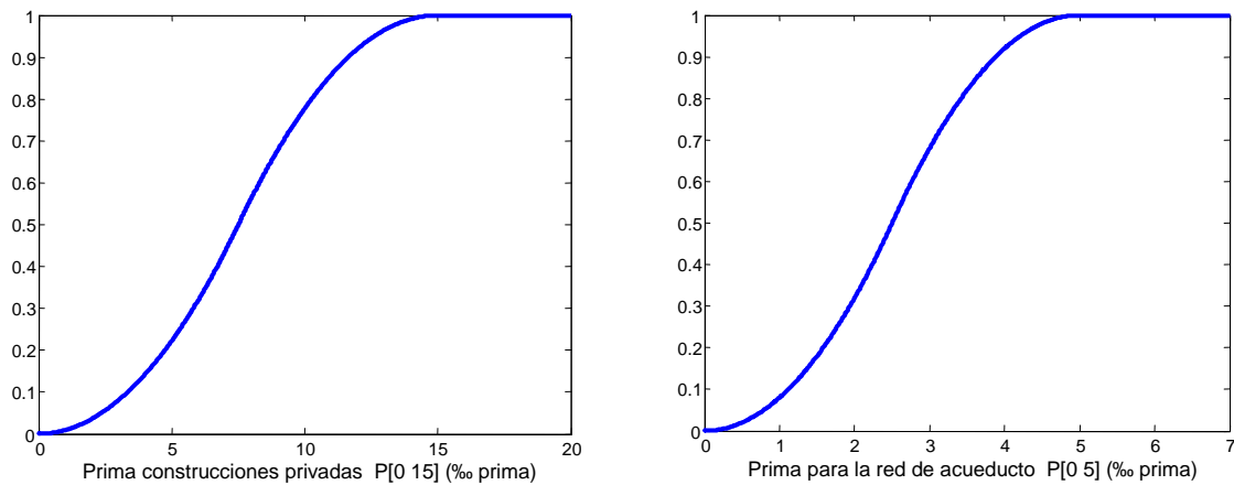
Figura 3-1 Funciones de transformación utilizadas
