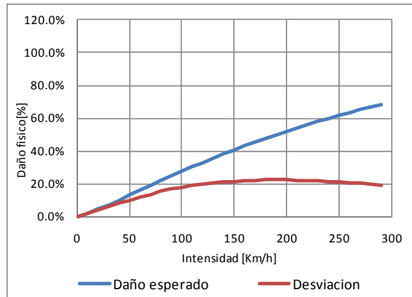
Figura 3-14 Función de vulnerabilidad ante viento, tipo constructivo MC-RCSM-4
