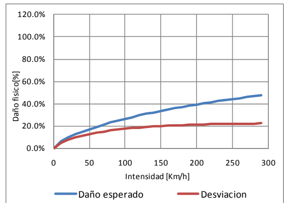
Figura 3-16 Función de vulnerabilidad ante viento, tipo constructivo R-SLFB-1
