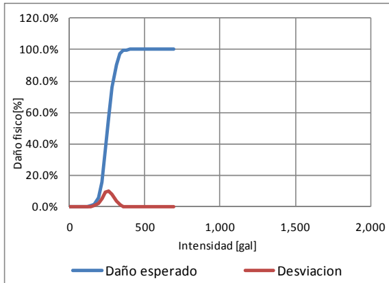
Figura 3-1 Función de vulnerabilidad sísmica, tipo constructivo A-SLSB-1
