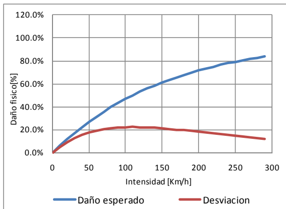
Figura 3-15 Función de vulnerabilidad ante viento, tipo constructivo W-FPFB-2
