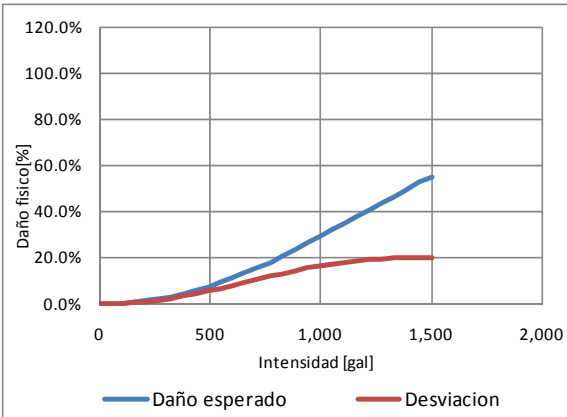
Figura 3-5 Función de vulnerabilidad sísmica, tipo constructivo PCR-RCSM-5
