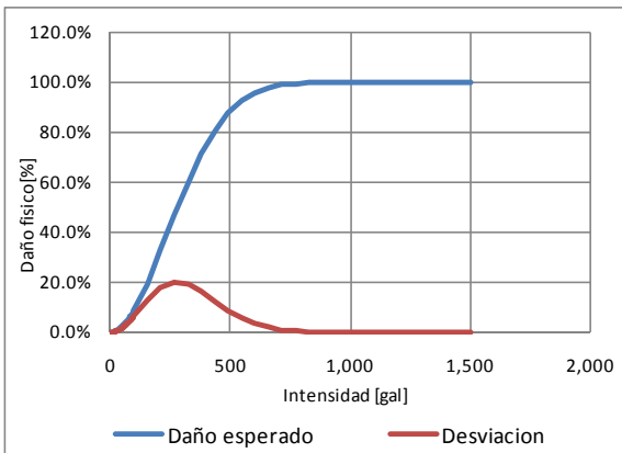
Figura 3-7 Función de vulnerabilidad sísmica, tipo constructivo W-FPFB-1
