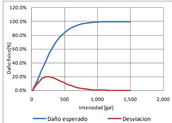
Figura 3-4 Función de vulnerabilidad sísmica, tipo constructivo B-SPFB-1
