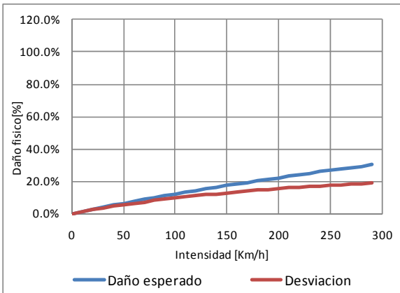
Figura 3-13 Función de vulnerabilidad ante viento a, tipo constructivo B-SPFB-1
