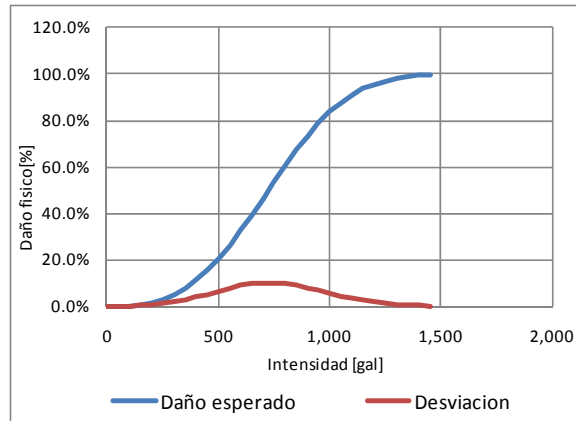
Figura 5-3 Función de vulnerabilidad para presas
