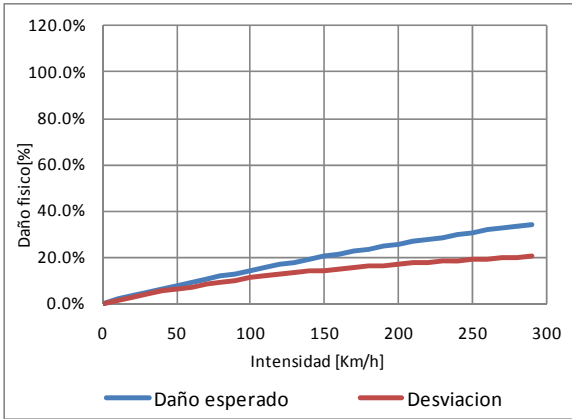
Figura 3-11 Función de vulnerabilidad ante viento, tipo constructivo PCR-RCSM-5
