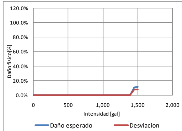
Figura 3-6 Función de vulnerabilidad sísmica, tipo constructivo MC-RCSM-4
