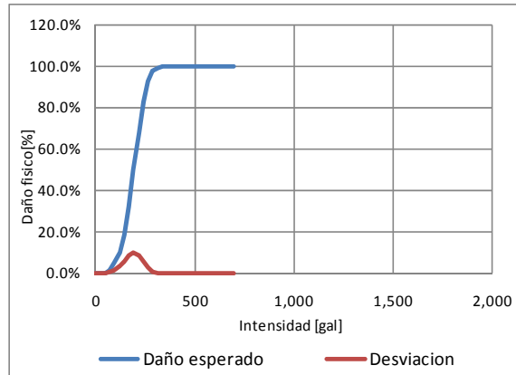
Figura 3-2 Función de vulnerabilidad sísmica tipo constructivo MS-FLSB-1
