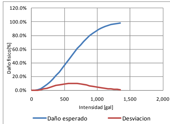
Figura 5-6 Función de vulnerabilidad para muelles
