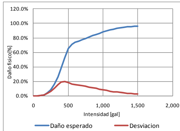
Figura 5-1 Función de vulnerabilidad para subestaciones eléctricas
