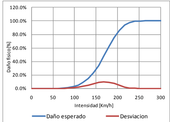
Figura 3-12 Función de vulnerabilidad ante viento, tipo constructivo MS-FLSB-1
