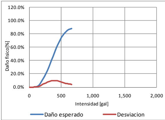
Figura 3-3 Función de vulnerabilidad sísmica, tipo constructivo MR-RLSB-2
