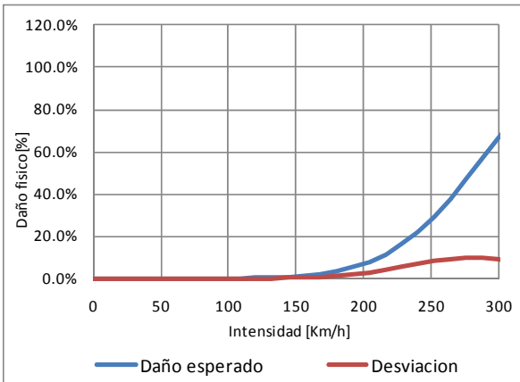
Figura 3-9 Función de vulnerabilidad ante viento, tipo constructivo A-SLSB-1
