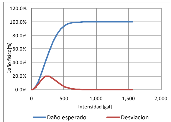
Figura 3-8 Función de vulnerabilidad sísmica, tipo constructivo R-SLFB-1
