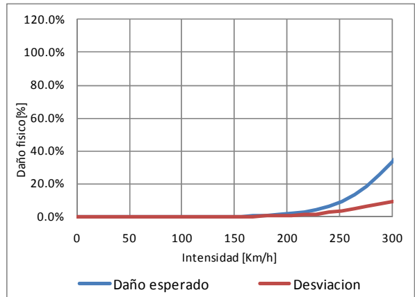
Figura 3-10 Función de vulnerabilidad ante viento, tipo constructivo MR-RLSB-2
