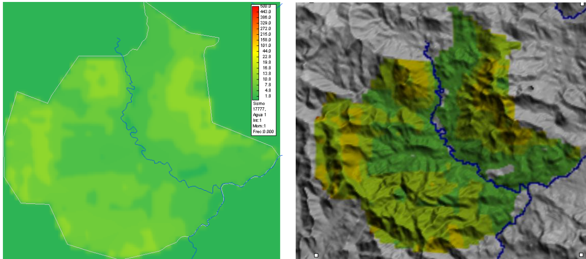
Figura 5-1 Mapa de amenaza por deslizamiento para el municipio de San Dionisio. Estado de suelo seco con sismo. Análisis método Mora Vahrson.
