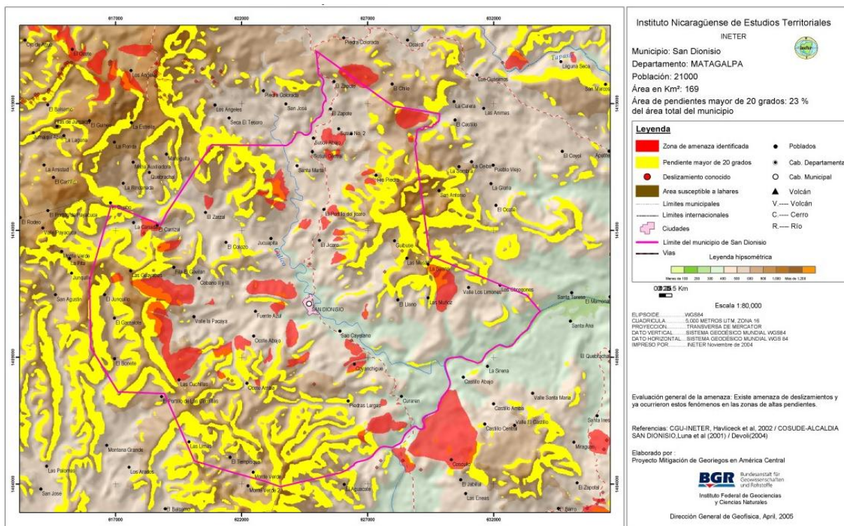
Figura 1-2 Evaluación general de amenaza. Municipio de San Dionisio. (Fuente: INETER)
