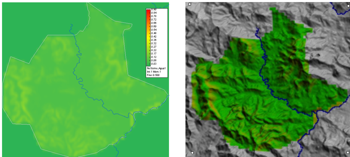
Figura 5-2 Mapa de amenaza por deslizamiento para el municipio de San Dionisio. Estado de suelo seco sin sismo. Análisis método de falla traslacional.
